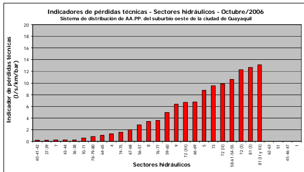
Figura 13. Indicadores de pérdidas técnicas de sectores hidráulicos para octubre del 2006.
