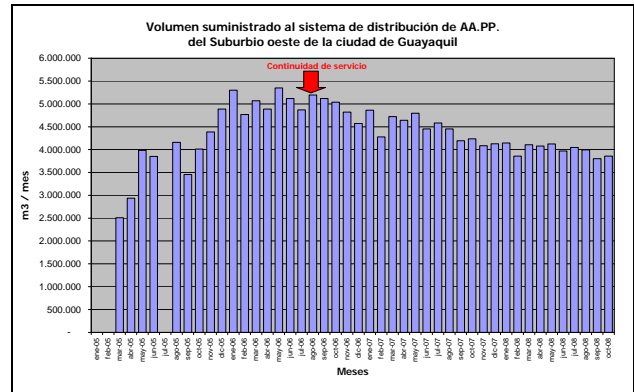
Figura 15. Volumen suministrado a la red de distribución entre marzo del 2005 y octubre del 2008.
