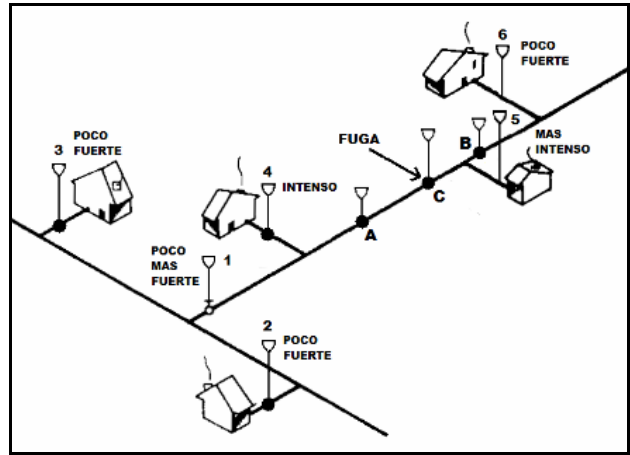
Figura 10. Esquema de prelocalización y localización de fugas no visibles con el empleo de geófonos.
