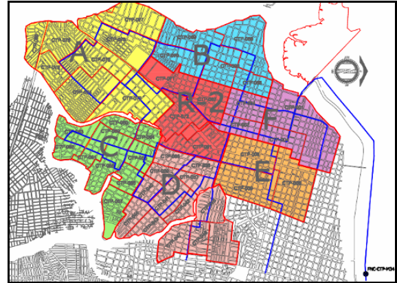
Figura 4. Macrosectores hidráulicos definidos en la red de distribución de AA.PP. del suburbio oeste de la ciudad de Guayaquil.
