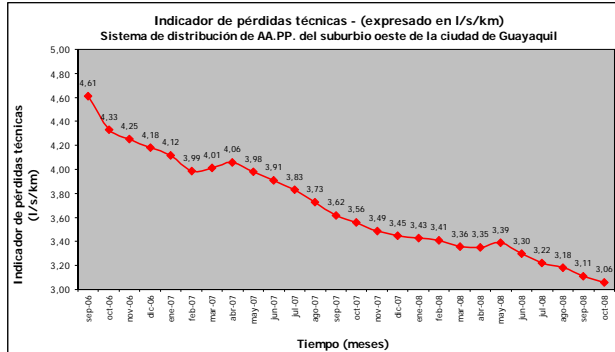
Figura 12. Indicador de pérdidas técnicas de la red de distribución de AA.PP. del suburbio oeste.
