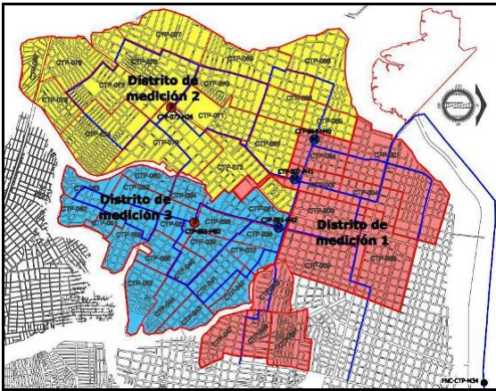
Figura 3. Distritos de medición en la red de distribución de AA.PP. del suburbio oeste de la ciudad de Guayaquil.
