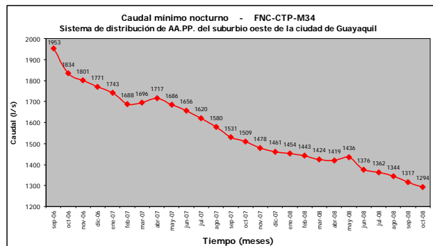
Figura 11. Caudal mínimo nocturno
