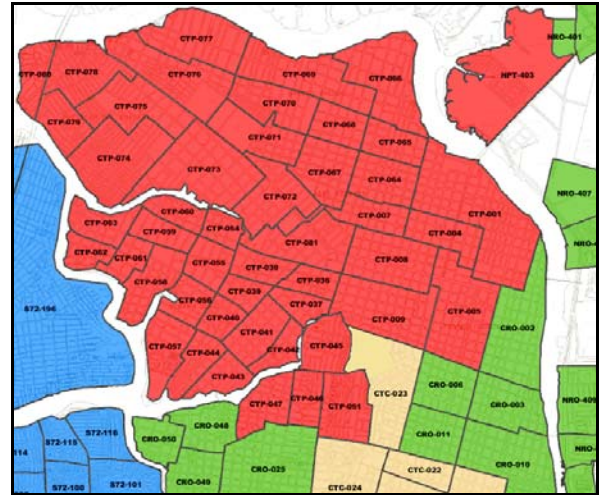
Figura 2. Sectorización hidráulica de la red de distribución de AA.PP. del suburbio oeste de la ciudad de Guayaquil
