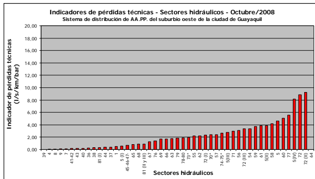
Figura 14. Indicadores de pérdidas técnicas de sectores hidráulicos para octubre del 2008.
