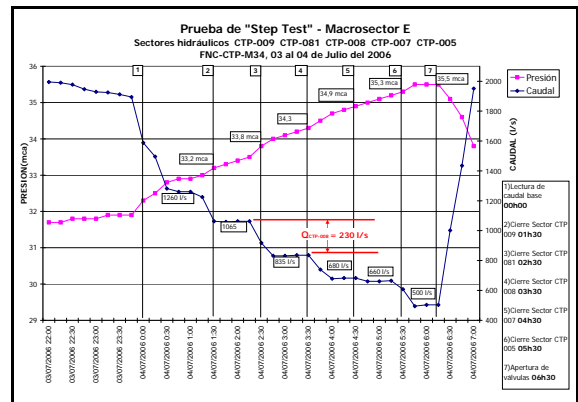
Figura 5. Informe gráfico de prueba de Step Test
