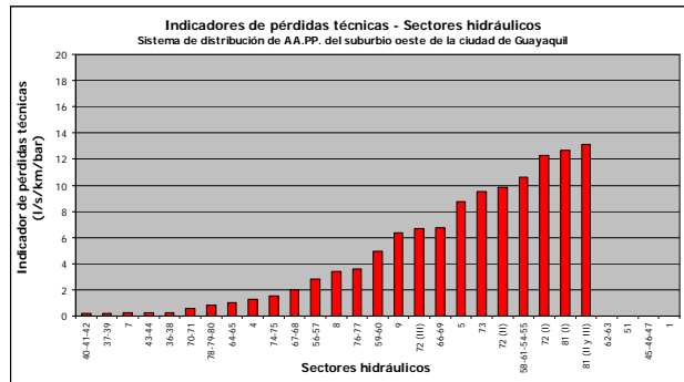
Figura 6. Gráfico de barras obtenido con valores de indicadores de pérdidas técnicas.
