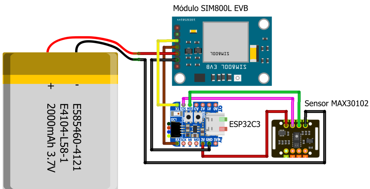
Figura 3.1: Diagrama del circuito
