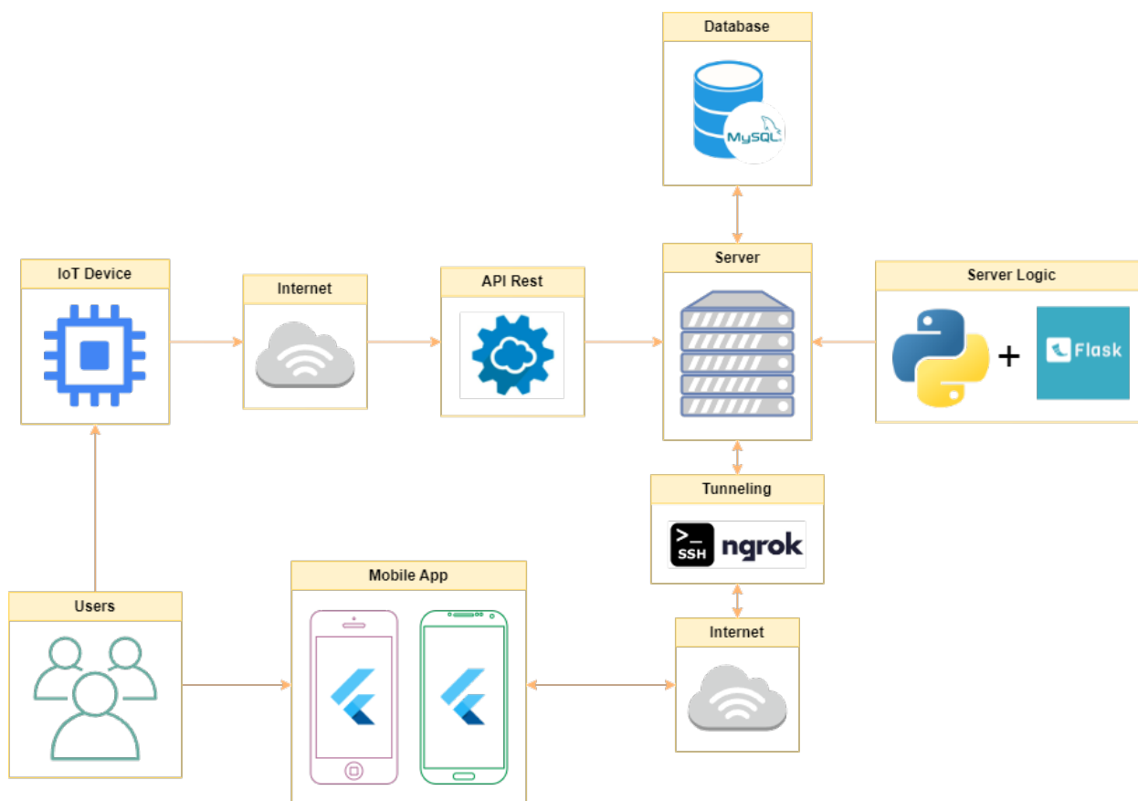
Figura 2.4: Diagrama de Arquitectura
