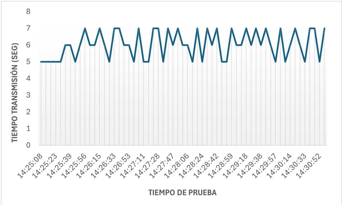
Figura 3.2: Gráfico Tiempo de Transmisión vs Tiempo de Prueba Operadora X
