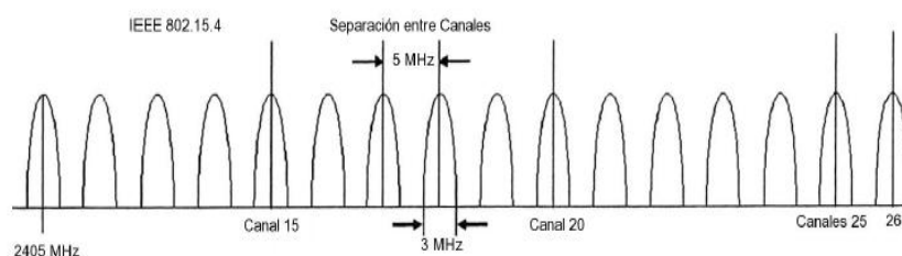
Figura C4 Canales disponibles de transmisión de módulos XBee [20]
